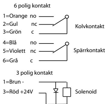
Kopplingschema för STEP 29 Silent™
