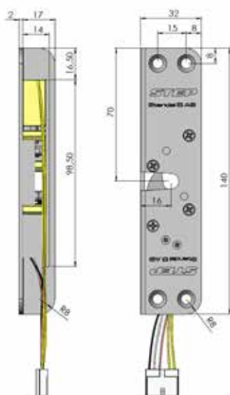
STEP 35 med vinklad stolpe
