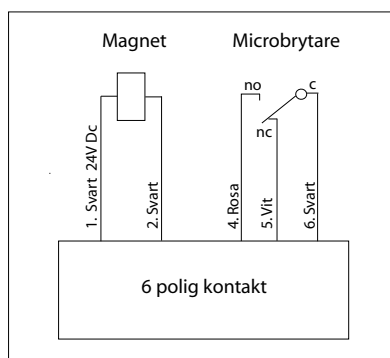
Kopplingsschema STEP 35
