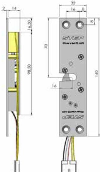
STEP 35 med plan stolpe
